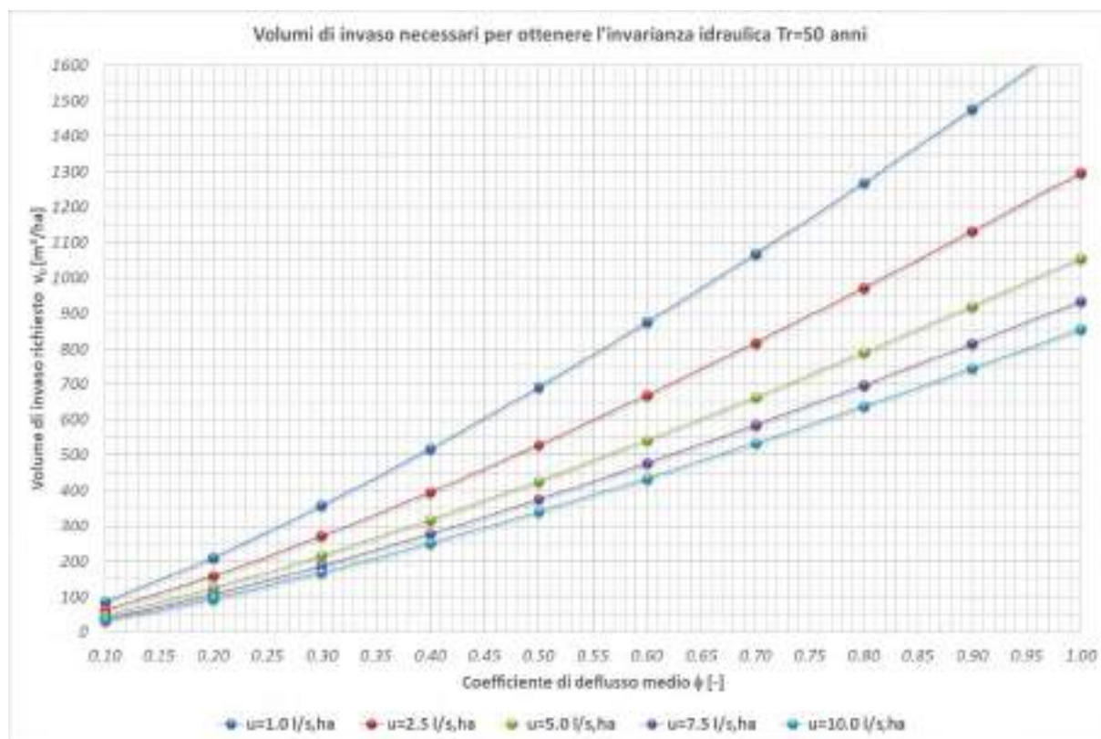
Fig. 6.1 - Volumi di invaso in m^3/ha necessari per ottenere l'invarianza idraulica per T_r=50 anni e CPP a 3 parametri a , b e c . Dalla Tabella è possibile ricavare i volumi di invaso specifico in funzione del coefficiente di afflusso medio f e del coefficiente udometrico massimo u , in uscita (rappresentato in vari colori nel grafico)
